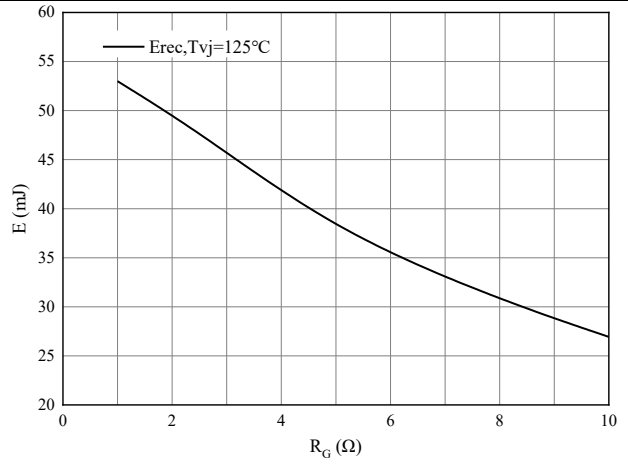
图 8. 开关损耗 二极管 Figure 8. Switching losses of Diode I_F=400A, V_{CE}=900V
