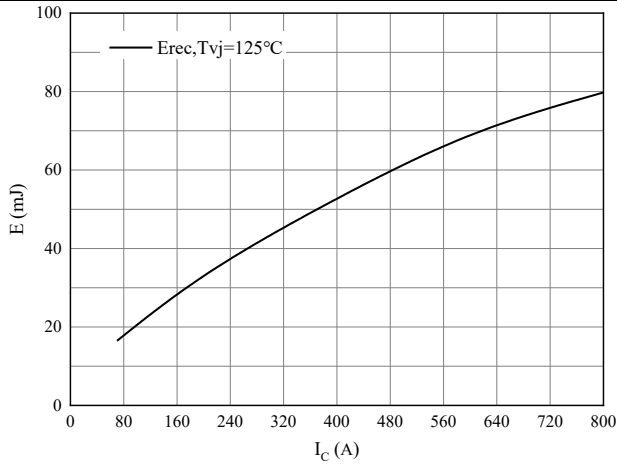
图 7. 开关损耗 二极管 Figure 7. Switching losses of Diode R_{Gon}=1\Omega, V_{CE}=900V
