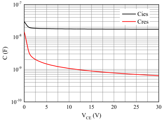
图 9. 电容特性
